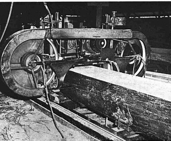
Gergaji membelah kayu2 balak yang di-gunakan dalam kilang papan.
