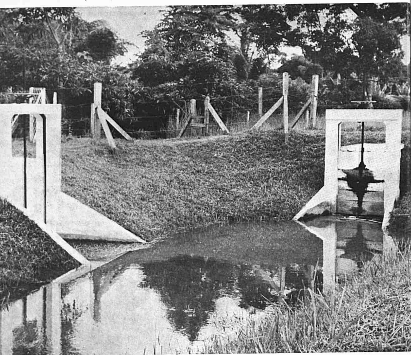
Pintu ayer di-Paya Kangsar, Jerantut.
